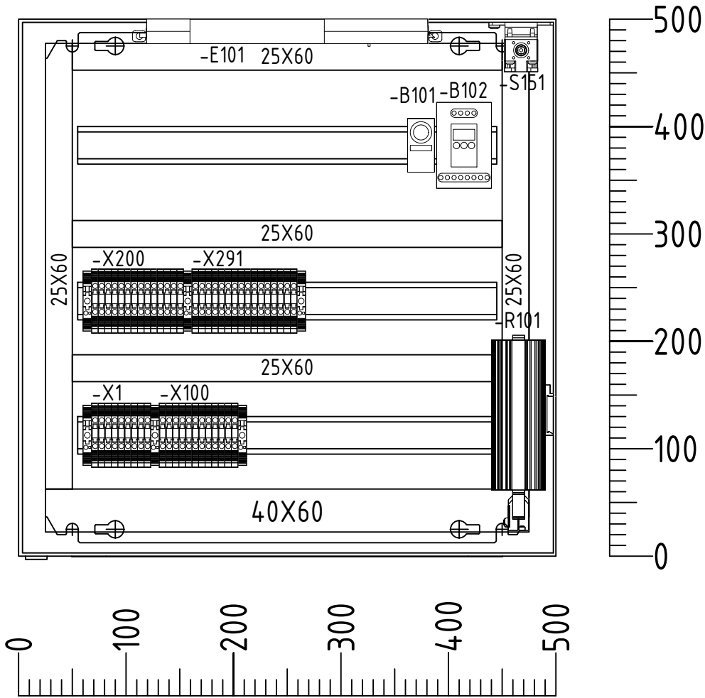
Prednji izgled bez vrata
