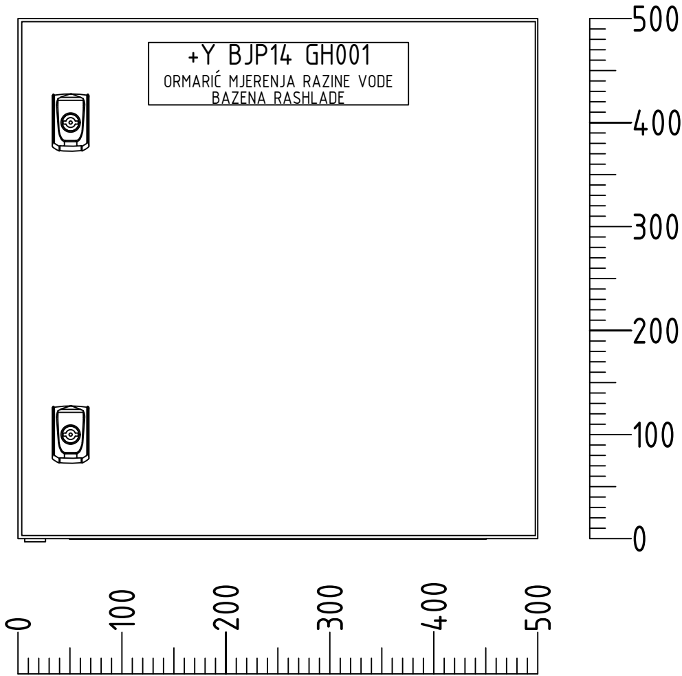
Prednji izgled s vratima
